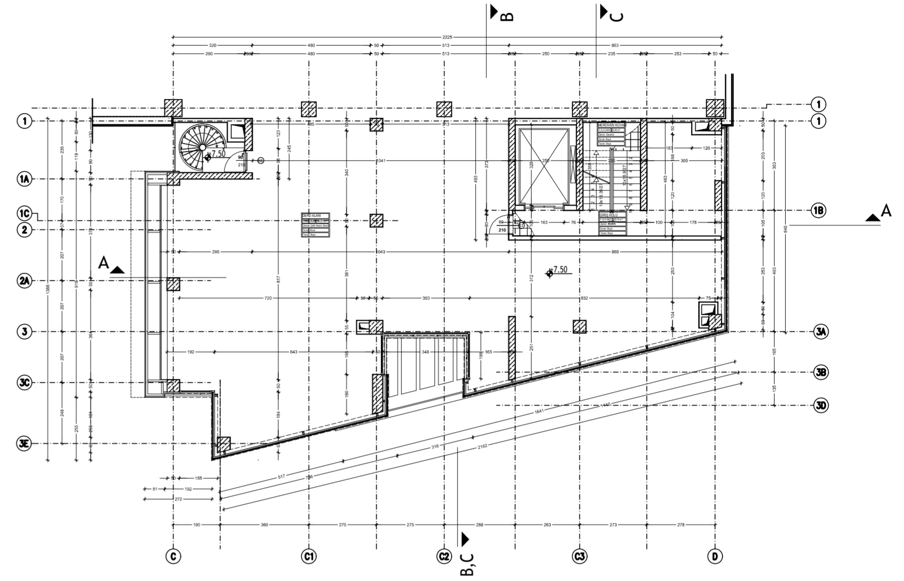
F, G, H BLOK TİP İDARİ BÖLÜM 2.NORMAL KAT PLANI
