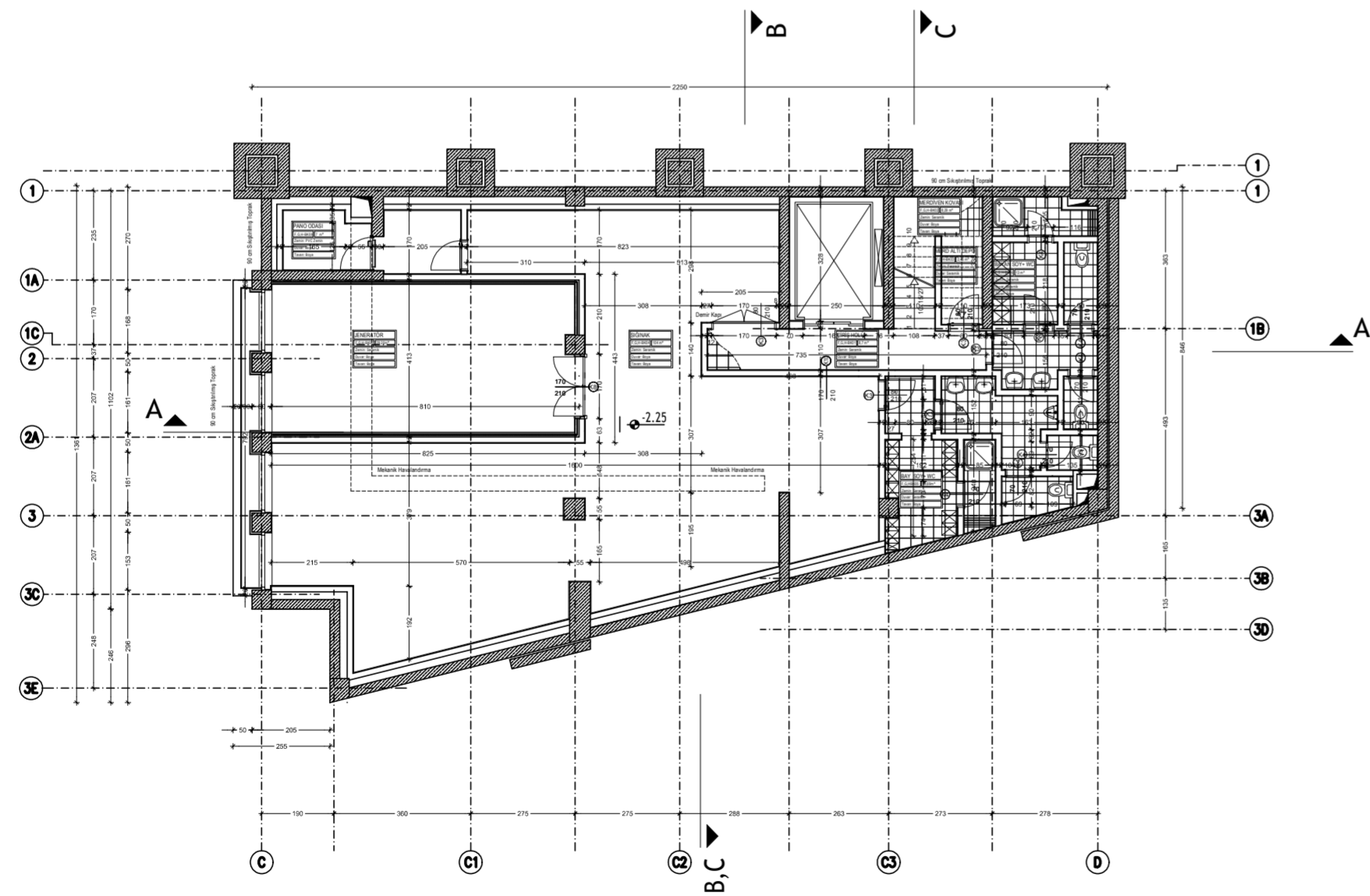
F, G, H BLOK TİP İDARİ BÖLÜM BODRUM KAT PLANI
