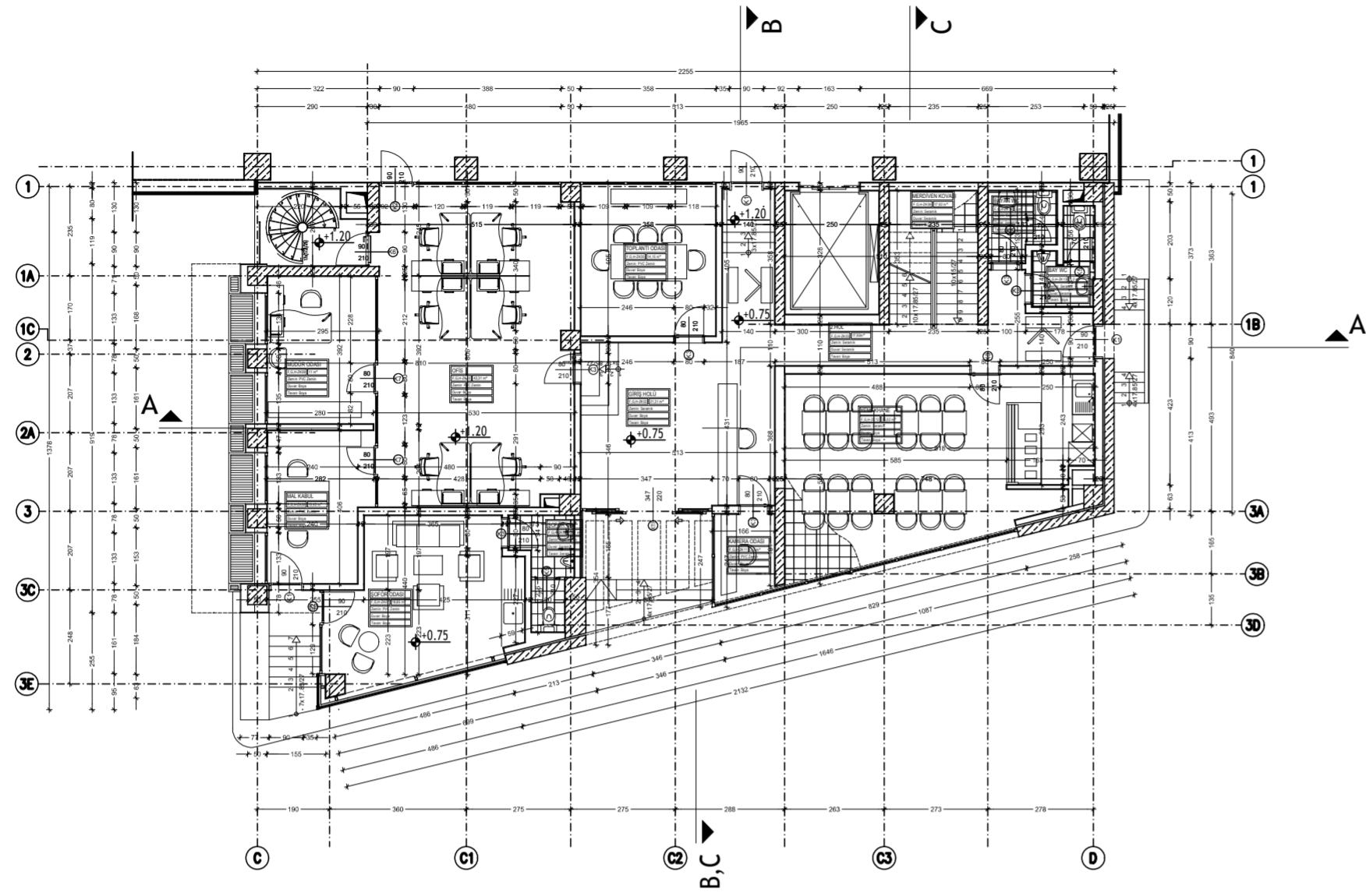
F, G, H BLOK TİP İDARİ BÖLÜM ZEMİN KAT PLANI
