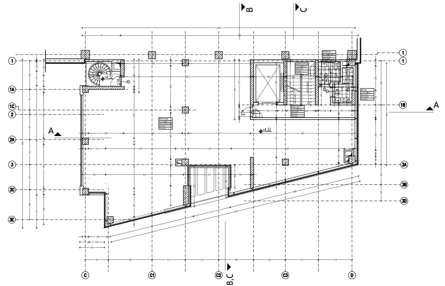
F, G, H BLOK TİP İDARİ BÖLÜM 1.NORMAL KAT PLANI
