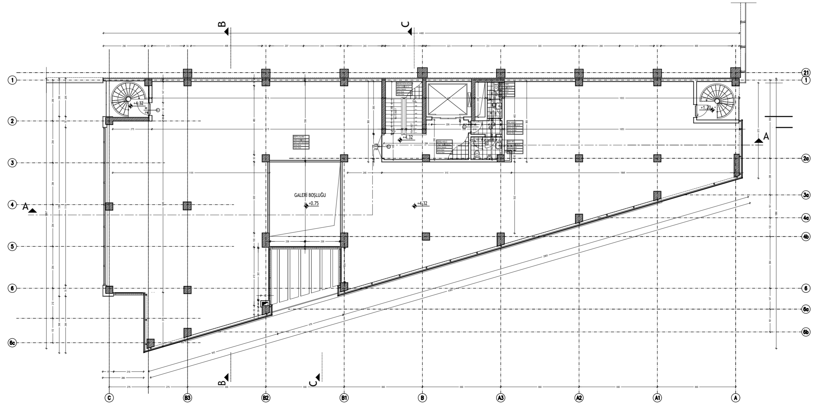
A, B, C, D BLOK TİP İDARİ BÖLÜM 2.NORMAL KAT PLANI
