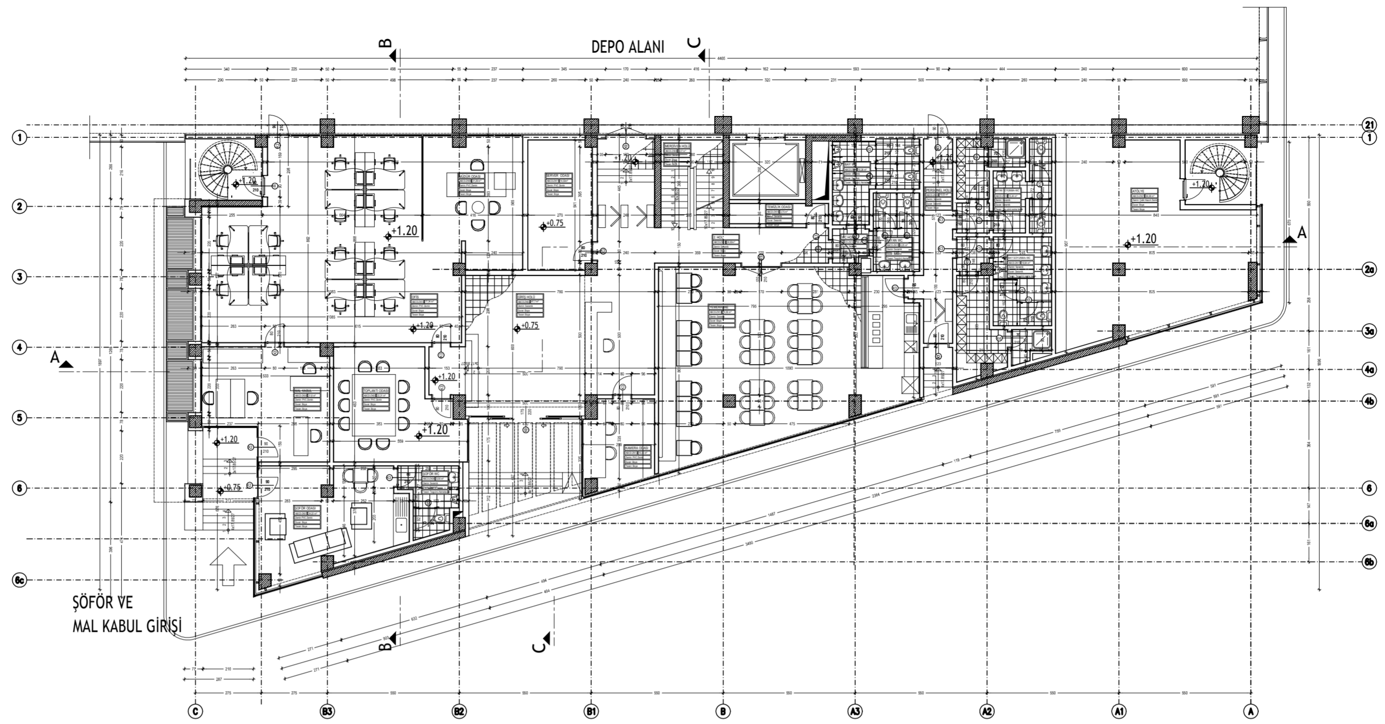
A, B, C, D BLOK TİP İDARİ BÖLÜM ZEMİN KAT PLANI
